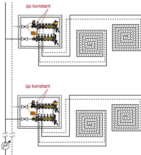
Steuerung \Delta p an Anlagen mit Verteilern
